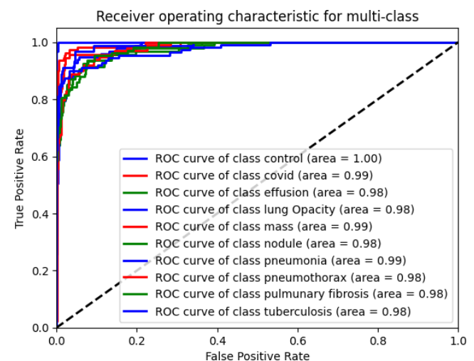
Fig. 2. ROC CNN
