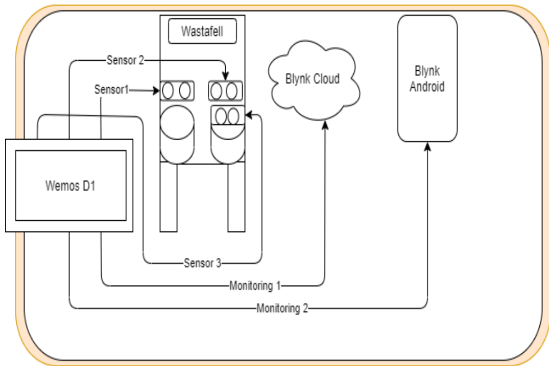
Gambar 2. Perancangan Interface Prototipe
