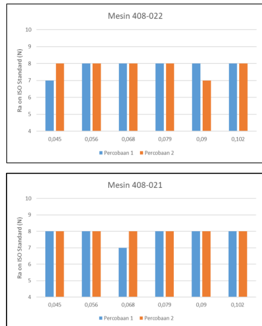
GAMBAR 9. Grafik pengaruh feeding terhadap nilai kekasaran menurut standard ISO (N) pada mesin 408-022 dan 408-021.
